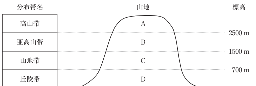
図1 日本の本州中部におけるバイオームと山地の標高の関係（模式図）
