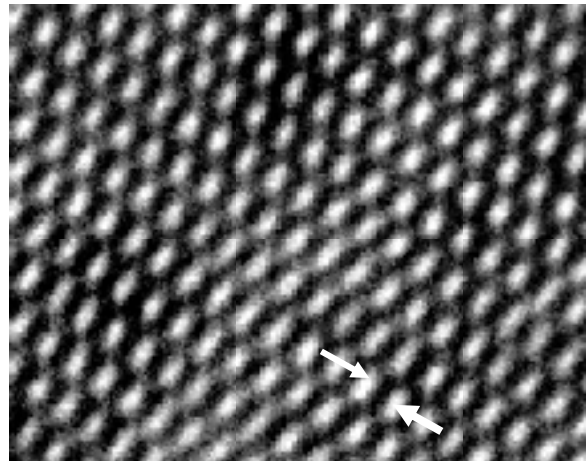
明るい点がチタン原子（矢印間隔 0.3 nm）
